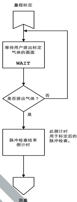
图 13 Xcel 脉冲技术设备的标定后脉冲检查
