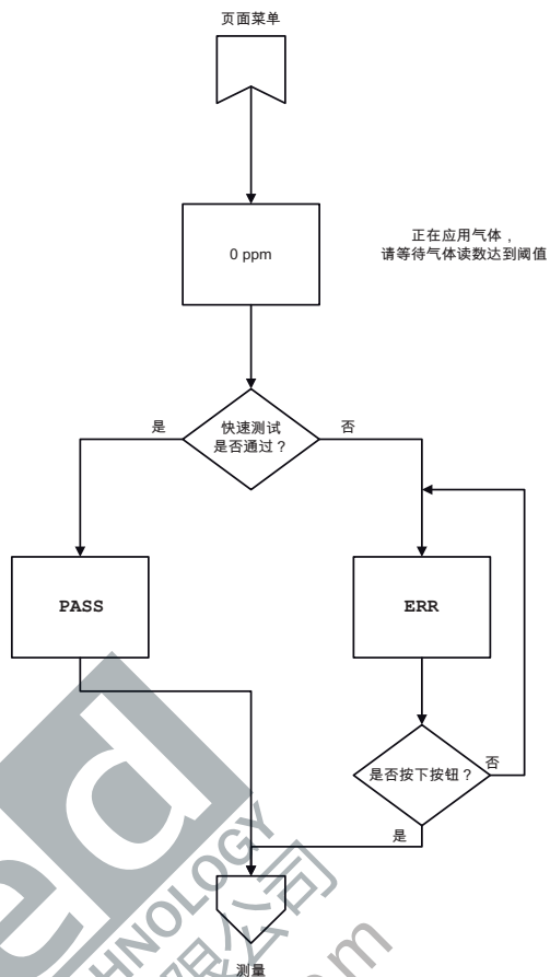
图 9 对未采用 XCell 脉冲技术的设备进行快速测试
